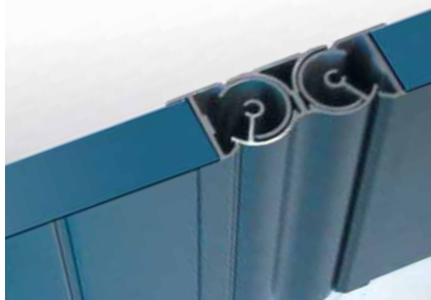
Panneaux sandwichs isolants de 40 mm. Double articulation anti-pince doigts pour portillon.
