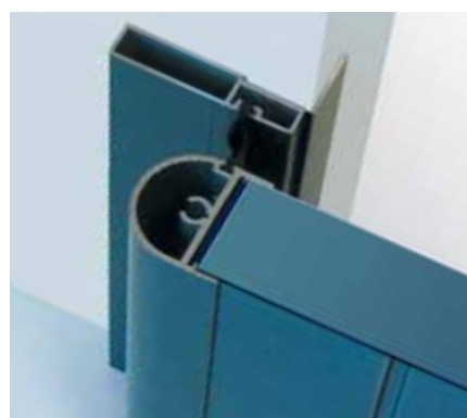
Joint lèvres sur le Précadre et sur la porte et cornière d'habillage avec maçonnerie.
