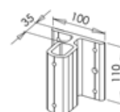
Embase pose en nez de dalle 100x110 Alu
